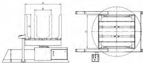
機械尺寸 (Machine Dimensions)
